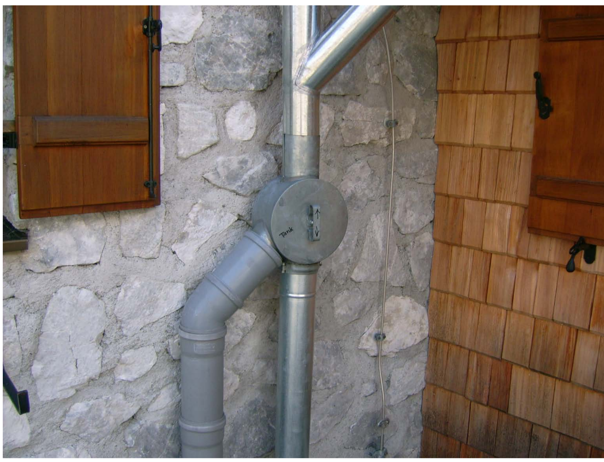
Regenwasserklappe
